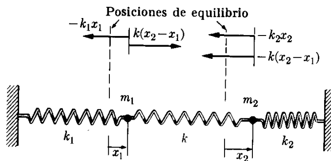
Fig. 12-27. Osciladores acoplados.
