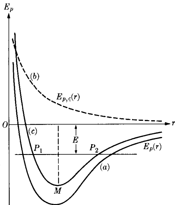
Fig. 8-22. Potencial intermolecular.
