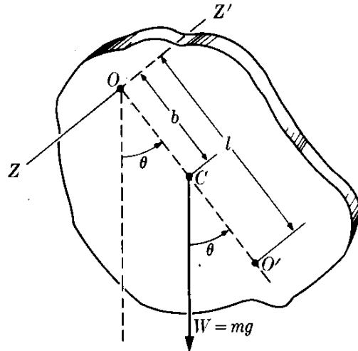
Fig. 12-11. Péndulo compuesto.
