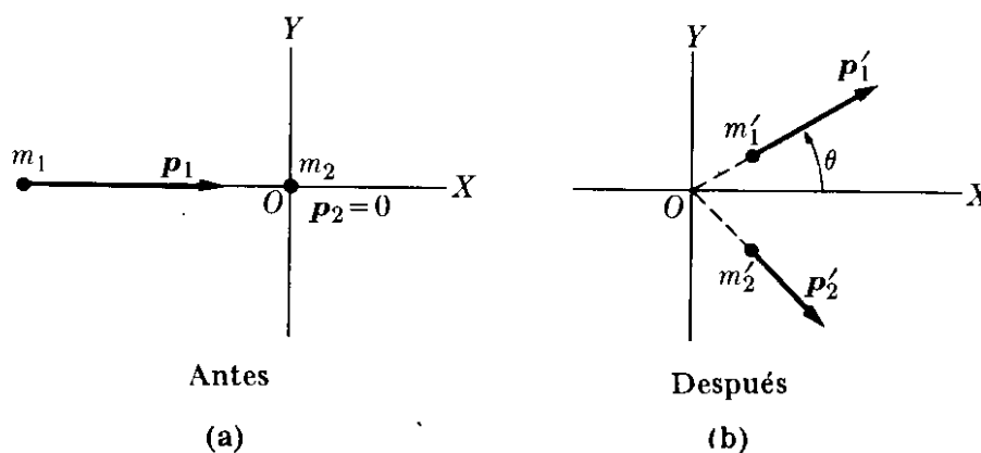
Fig. 9-12. Relación entre los momentos relativos al sistema- L antes y después del choque.
