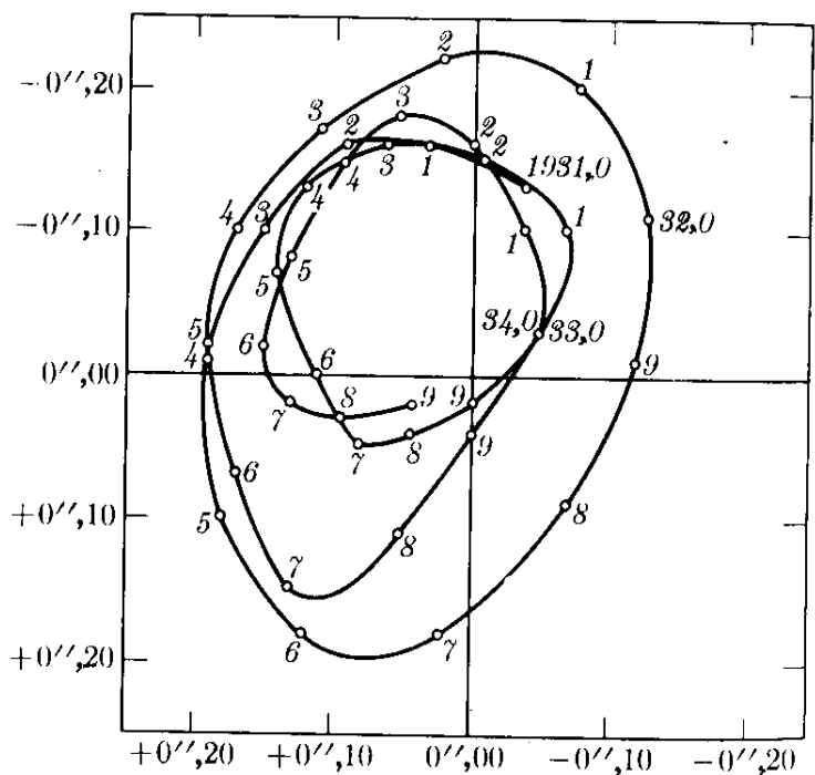
Fig. 10-19. Polhode del eje de rotación de la tierra en el periodo 1931-1935.
