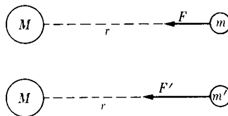
Fig. 13-5. Método de comparación de dos masas m y m' mediante su interacción gravitacional con una tercera masa M .
