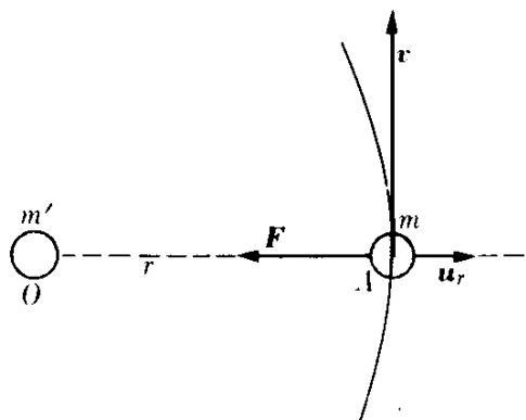
Fig. 13-6. La atracción gravitacional de m' sobre m es opuesta al vector unitario \mathbf{u}_r alejándose de m' .
