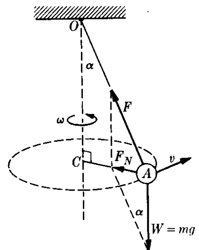
Fig. 7-18. Péndulo cónico.
